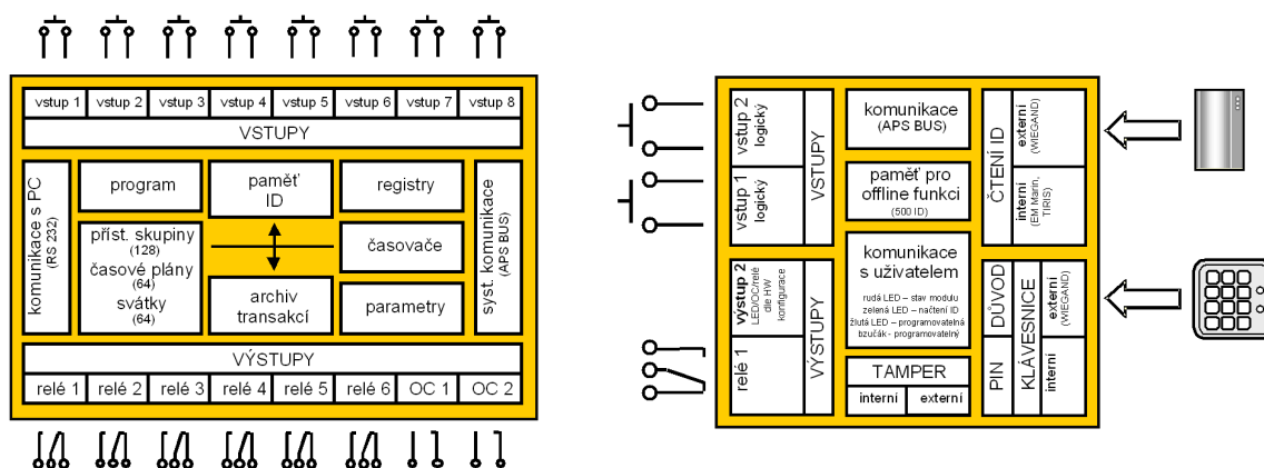
Obr. 3.2: Blokovaná schémata řídicího a síťového modulu
