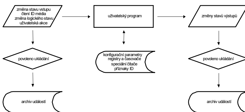
Obr. 3.5: Postup zpracování události
