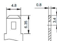
Terminal (F1)
